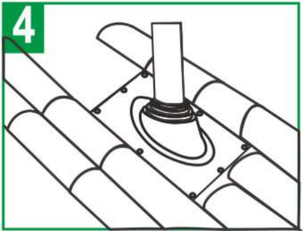
Установите и закрепите саморезами уплотнитель на кровлю
