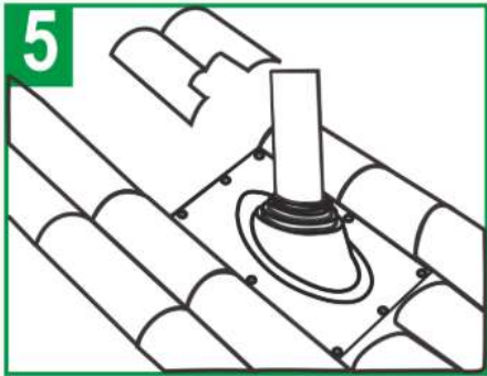
Вырежьте верхние элементы кровли по форме уплотнителя. Нижняя часть алюминиевого фланца должна остаться сверху кровли
