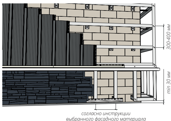
Рисунок 11. НФС с цоколем
