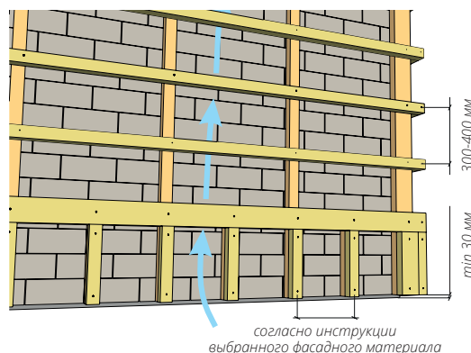
Рисунок 12. Деревянная обрешетка с цоколем
