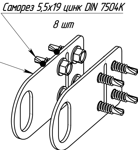
Проушина (в сборе)
