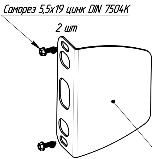
Ответная планка MEDIUM (в сборе)
