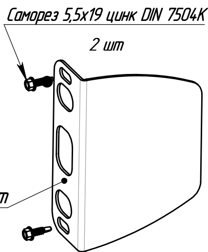
Ответная планка MEDIUM (в сборе)
