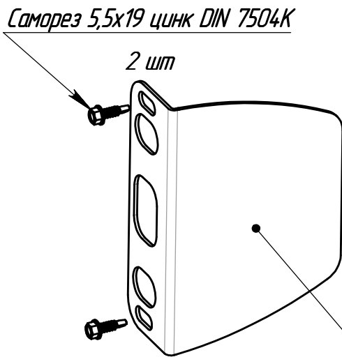
Ответная планка MEDIUM (в сборе)
