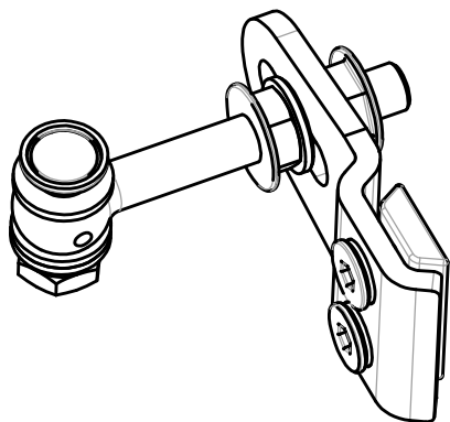
Петля GBMU4D12-Z-90-02-50 4 шт.
